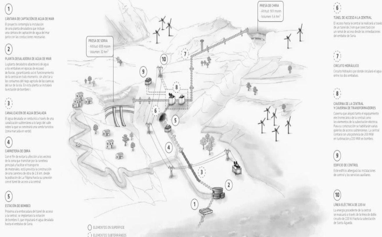
Ilustración 1 Esquema del Complejo Chira Soria. REE.
